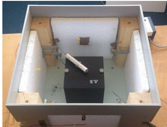
Obr. 2 Pohľad do vnútra boxu s inštalovanými termočlánkami
